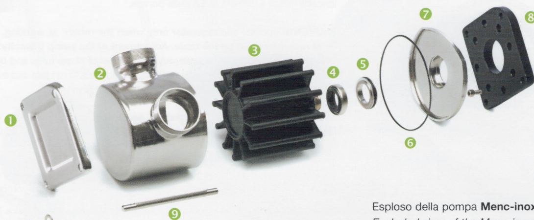
Esploso della pompa Menc-inox 50 Exploded view of the Menc-inox 50 pump Dessin des détails de la pompe Menc-inox 50
