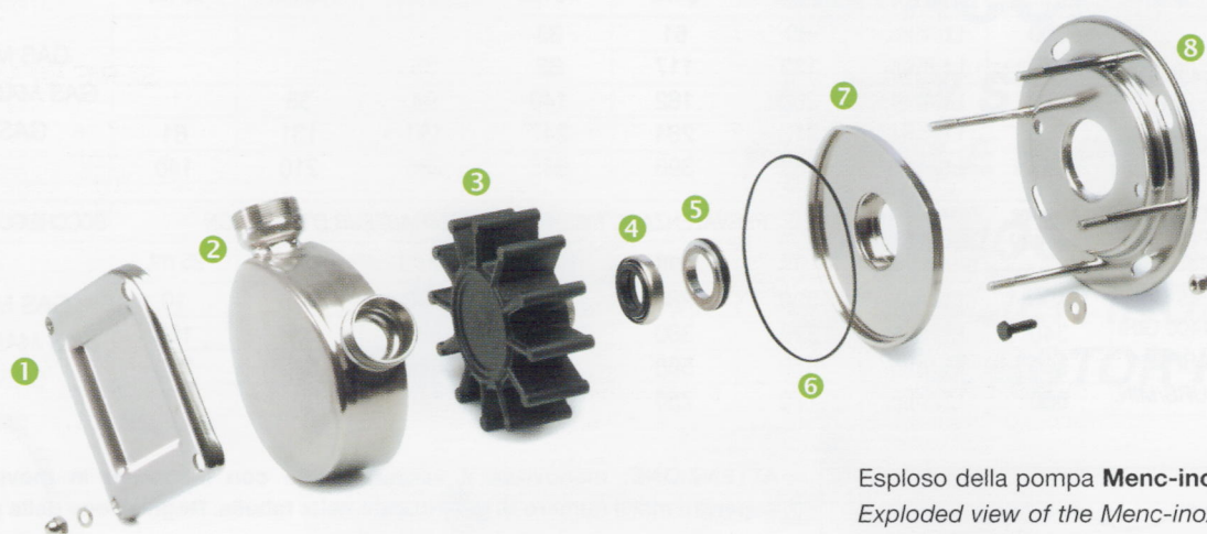
Esploso della pompa Menc-inox 40 Exploded view of the Menc-inox 40 pump Dessin des détails de la pompe Menc-inox 40
